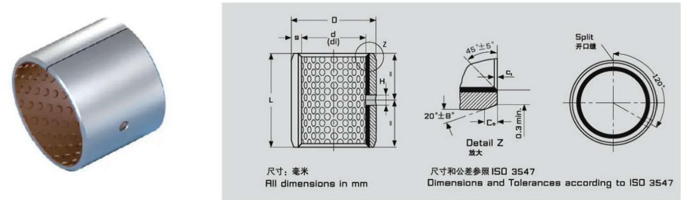
内外倒角尺寸表 Inside & Outside Chamfers
